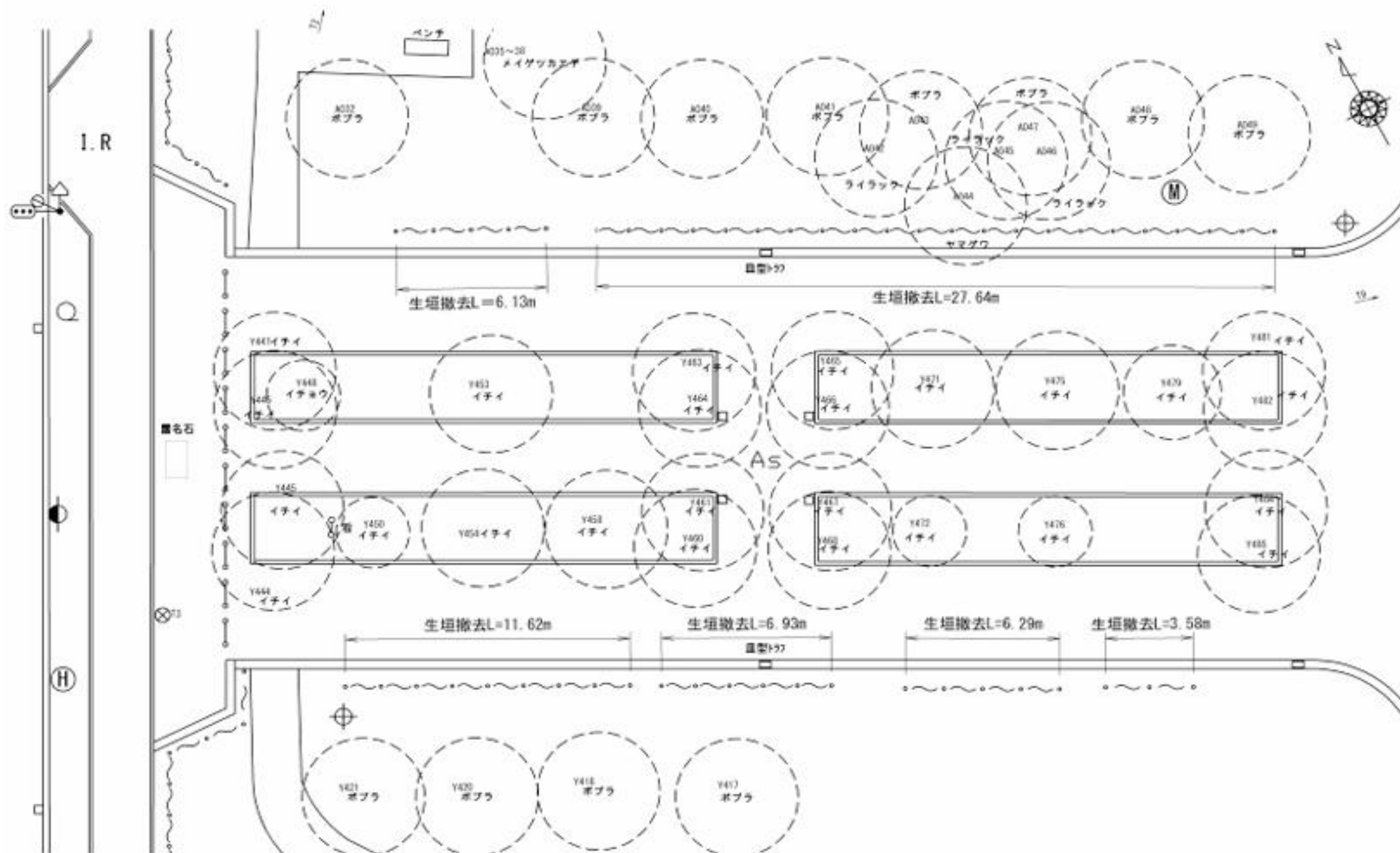
メインエントランス伐採抜根平面図 S=1:100
